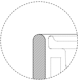
DETTAGLIO PROFILO BORDO SUPERIORE, VERSIONE LACCATA / TOP EDGE PROFILE DETAIL, LACQUERED VERSION
