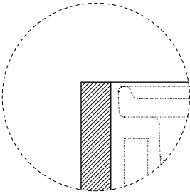
DETTAGLIO PROFILO BORDO SUPERIORE, VERSIONE IN ESSENZA / TOP EDGE PROFILE DETAIL, WOODEN FINISH VERSION
