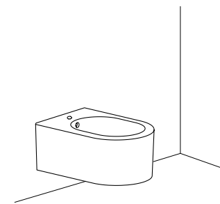
BIDET SOSPESO OTIS MONOFORO Otis wall-hung bidet with 1 hole cm 56 x 38,5 x 25 h
