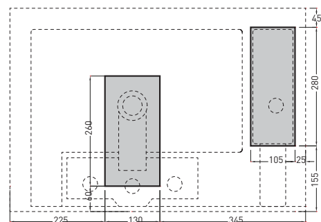
FORO SU PIANO OPZIONE 2 (RUBINETTO LATERALE) ON TOP HOLE OPTION 2 (SIDE TAP)
