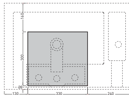
FORO SU PIANO OPZIONE 1 ON TOP HOLE OPTION 1
