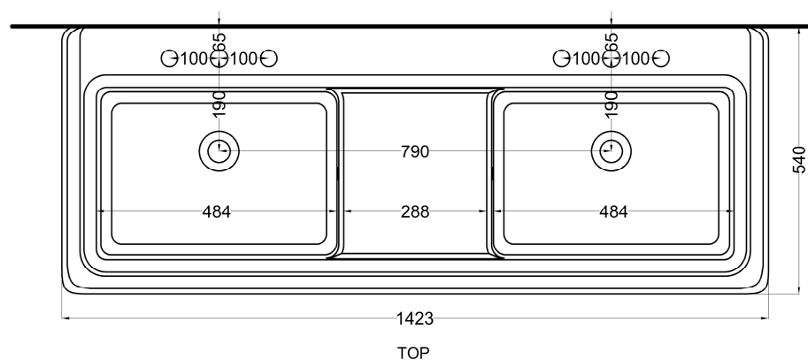
TOP
